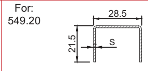
TRE 18 S=1.2mm S=1.5mm
