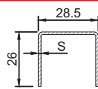
TRE 01 S=0.8mm S=1.2mm S=1.5mm S=2.0mm
